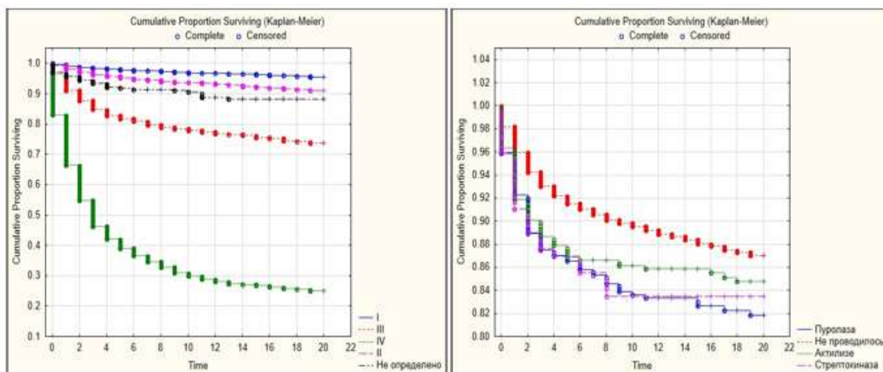
Рисунок 8 - Метод Каплана-Мейера: KILLIP (слева) и ТЛТ (справа)
