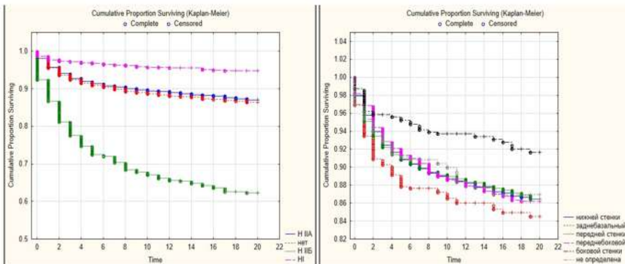
Рисунок 7- Метод Каплана-Мейера: ХСН (слева) и Локализация (справа)
