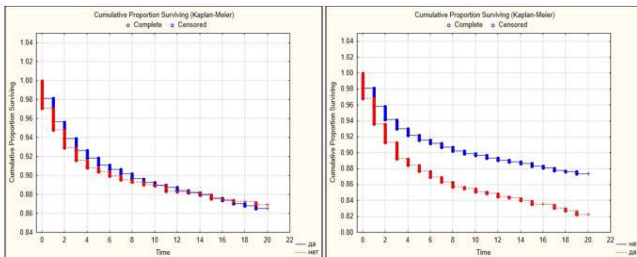
Рисунок 4. Метод Каплана-Мейера: АГ (слева) и ИМ (справа)
