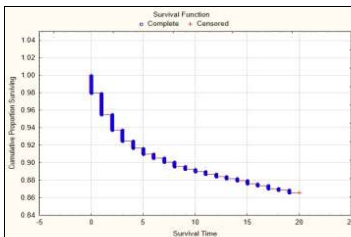
Рисунок 1 - График функции выживания
